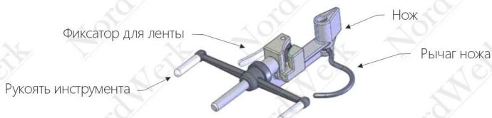
Рисунок 1 - Инструмент для натяжения и резки бандажной ленты
